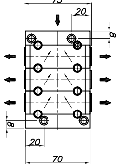
PROGRESIVO 6 SALIDAS
