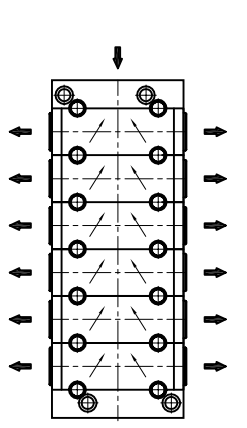
PROGRESIVO 12 SALIDAS
