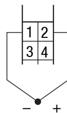
T/C Input
