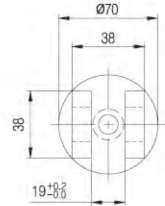
Rod Clevis (LA85-RC)
