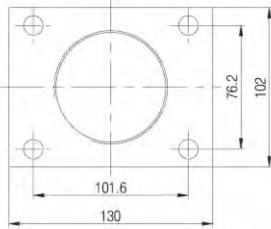
Rectangular Flange (LA85-RF)
