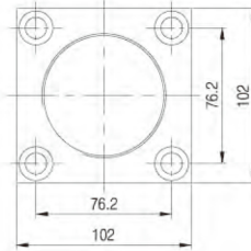
Square Flange (LA85-SF)
